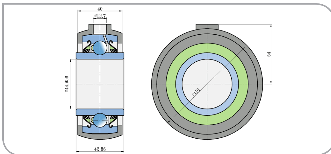
Rozměry/Dimensions (mm)
