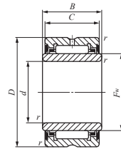
NA49...UU
