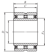
GBRI...UU
