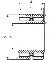
GTRI
