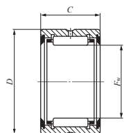
BR ... UU
