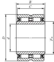
GBRI...UU
