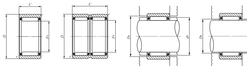
RNAF
