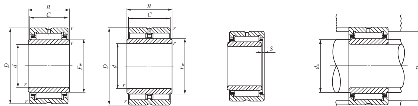
TRI
