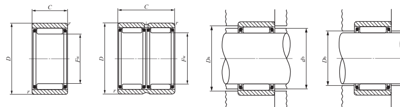
RNAF
