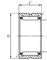
RNA49 RNA48
