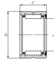
BR ... U
