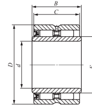
GBRI...U
