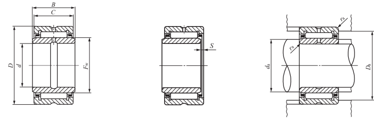
BRI
