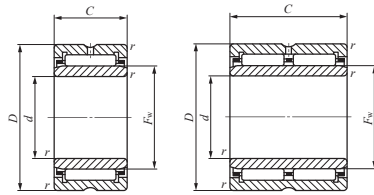
NA49 TAFI
