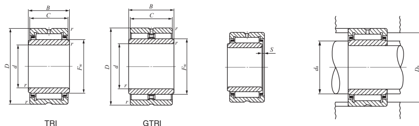
TRI
