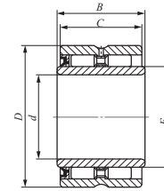
GBRI...U
