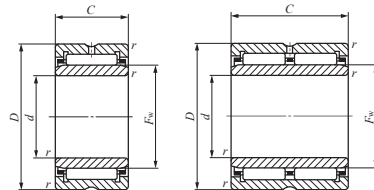
NA49 TAFI
