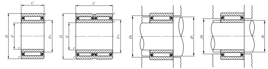
NAF
