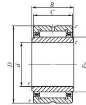
TRI
