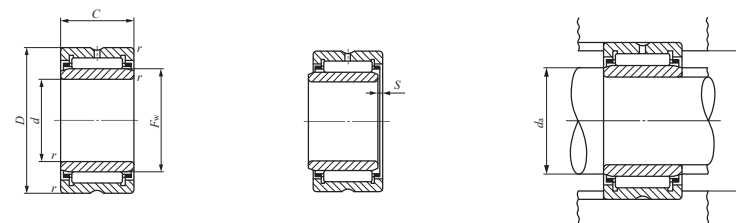
NA49 NA48
