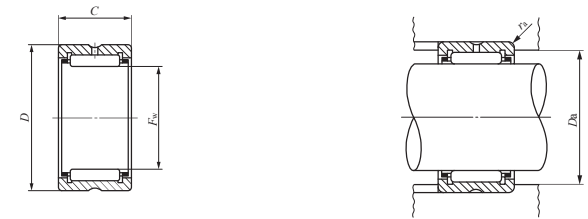
BR
