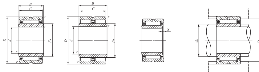
TRI
