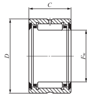
BR ... UU
