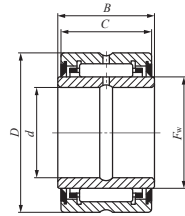
BRI ... UU
