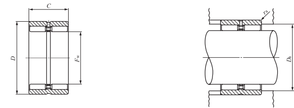
GBR
