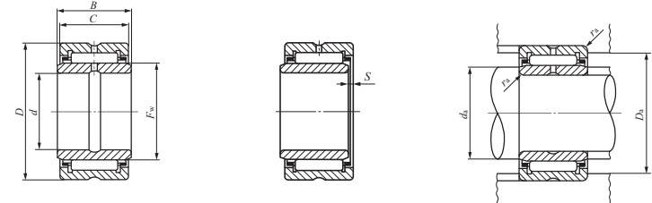
BRI
