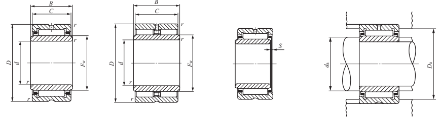
TRI
