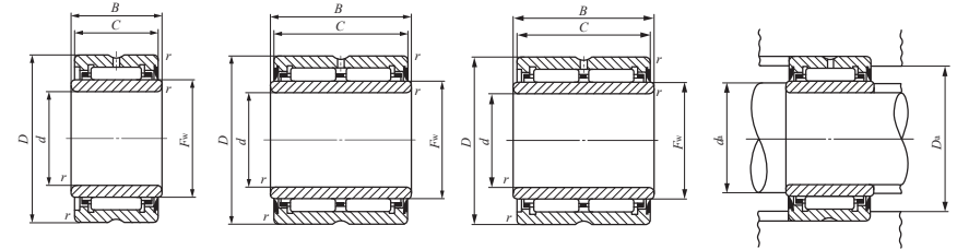
NA49...U
