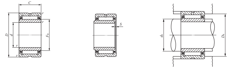
NA49 NA48
