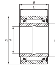
BRI ... U
