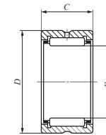
BR
