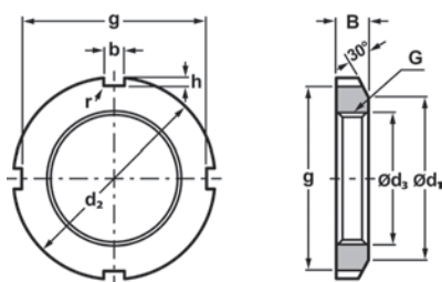
Matice s podložkou od AN05/KM05 po AN40/KM40
