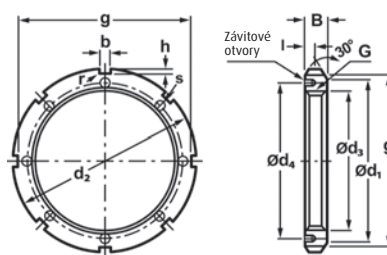
Matice s pojistnou vložkou od AN44/HM44T
