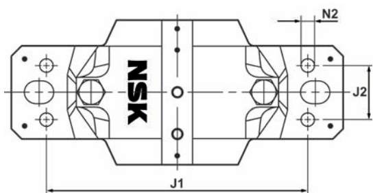
Doporučené rozměry pro 4 otvory upevňovacích šroubů (mm)
