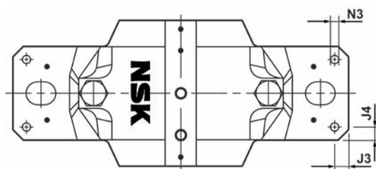
Doporučené rozměry pro otvory pro pojišťovací kolíky (mm)
