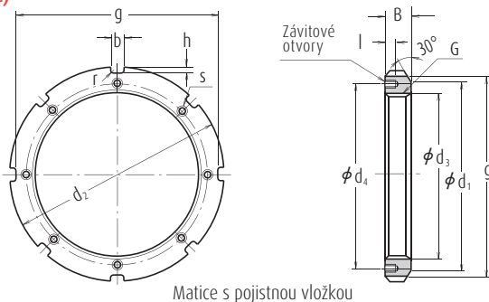
Matice s pojistnou vložkou
