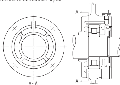
Obr. 12.1 Kombinace děleného zásobníku maziva a výstupního ventilu
