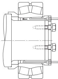
Obr. 14.7 Montáž na speciální pouzdro pomocí tlakového oleje
