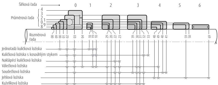
Obr. 3.1 Rozměrové řady radiálních ložisek
