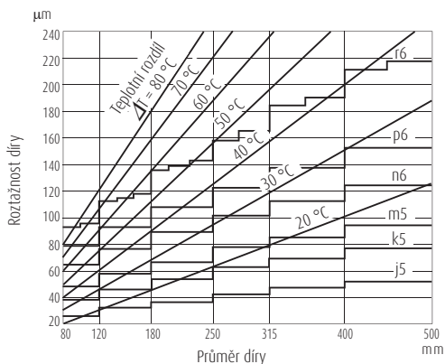
Obr. 14.3 Teplota a tepelná roztažnost vnitřního kroužku
