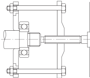
Obr. 14.13 Demontáž vnitřního kroužku použitím stahováků (1)
