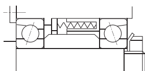
Obr. 10.2 Předpětí konstantní silou
