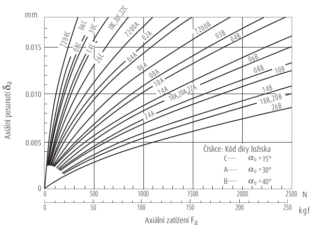
Obr. 15.3 Axialní zatížení a axialní posunutí kuličkových ložisek s kosohylným stykem
