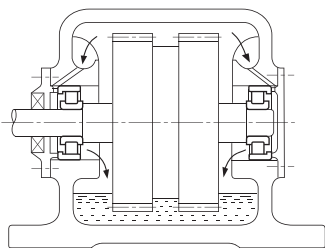
Obr. 12.6 Mazání rozstříkem
