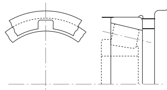
Obr. 14.11 Demontážní drážka
