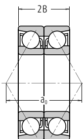
Zády k sobě - do "0" DB
