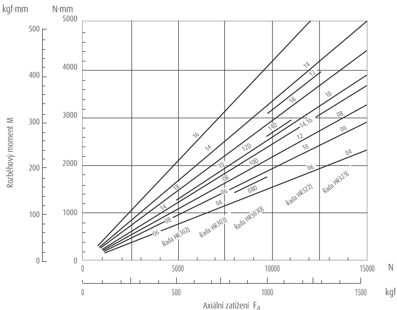
Obr. 15.10 Vztah mezi axiálním zatížením a rozběhovým momentem kuželikových ložisek
