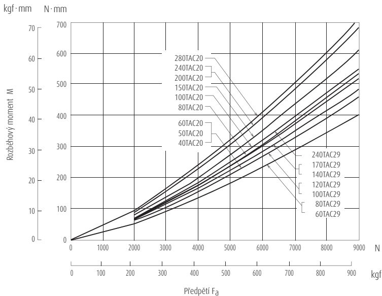
Obr. 15.12 Předpětí a rozběhový moment pro obousměrná axiální kuličková ložiska s kosohýlným stykem
