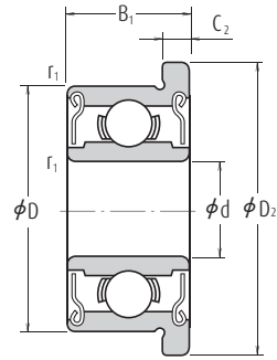
Zakrytá ZZ · ZZ1
