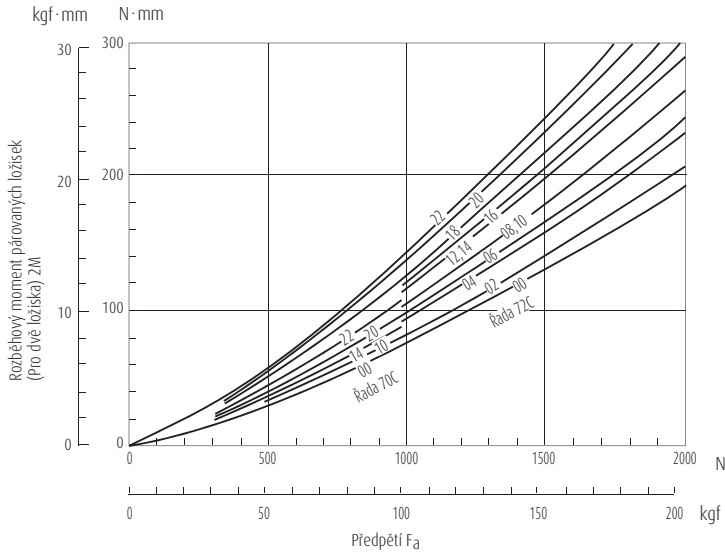
Obr. 15.11 Předpětí a rozběhový moment pro uspořádání kuličkových ložisek s kosohýlným stykem čely k sobě - do "X", nebo zády k sobě - do "O" ( \alpha = 15^\circ )
