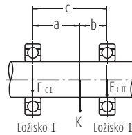
Obr. 5.5 Rozložení radiálního zatížení (1)
