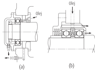
Obr. 12.8 Mazání vstříkovaným olejem
