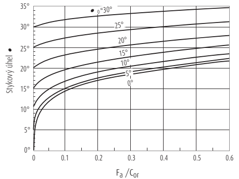
Obr. 15.1 F_a/C_{Or} a stykový úhel jednořadých kuličkových ložisek a kuličkových ložisek s kosoúhlým stykem
