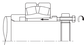
Obr. 14.5 Montáž na stahovací pouzdro
