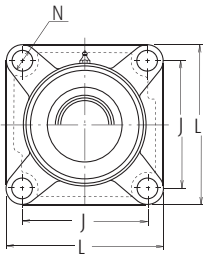
Jednotka s plechovým krytem Otevřený konec Z-UCF--D1 Uzavřený konec ZM-UCF--D1
