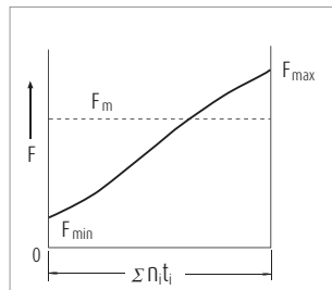
Obr. 5.8 Plynulé změny zátěže
