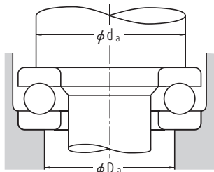
Obr. 11.3 Průměry podpůrných ploch axiálních kuličkových ložisek
