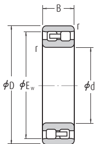
NN Válcová díra
