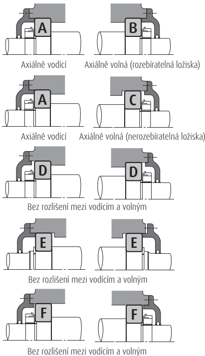
Obr. 4.1 Uspořádání ložisek
