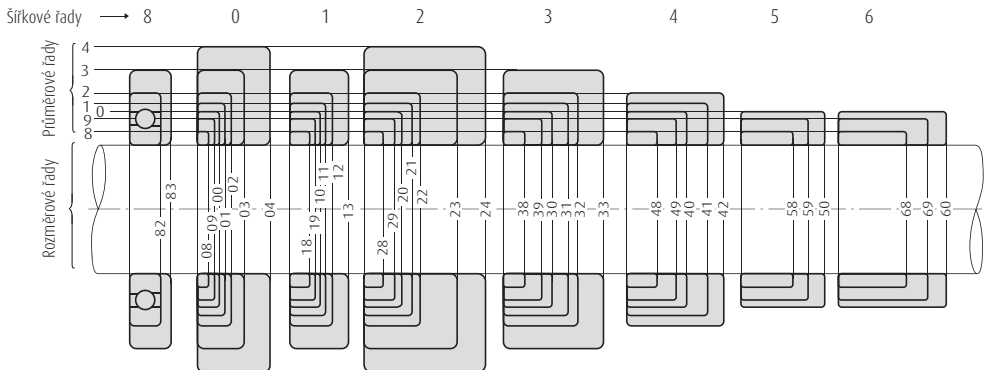
Fig. 7.6 Porovnání rozměrů průřezu radiálních ložisek (kromě kuželíkových ložisek) pro různé rozměrové řady
