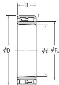
NNU Kruželová díra
