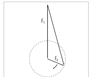
Obr. 5.10 Obvodové zatížení a statické zatížení
