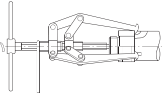
Obr. 14.14 Demontáž vnitřního kroužku použitím stahováků (2)
