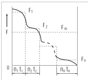
Obr. 5.7 Inkrementální (postupně) změny zátěže
