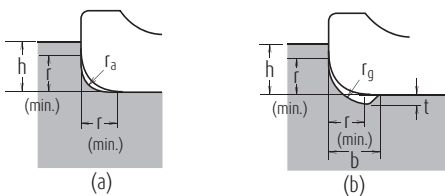
Obr. 11.2 Rozměry zápichů a opěrná výška
