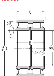
Bez pojistného kroužku
