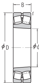
Kružlová díra
